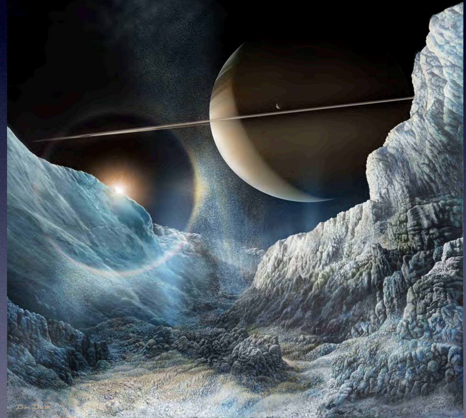
ENCELADUS
