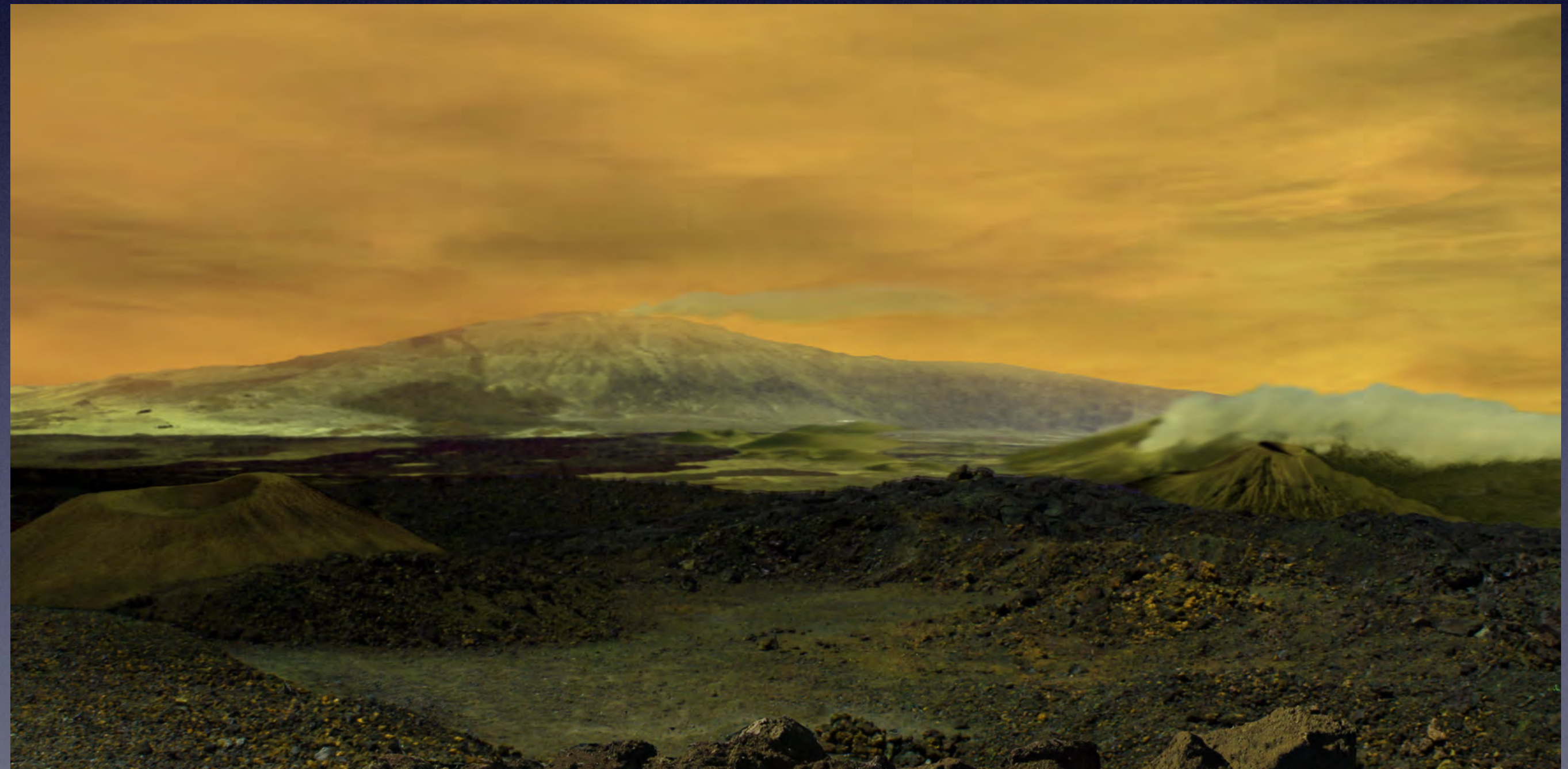
MAAT MONS
