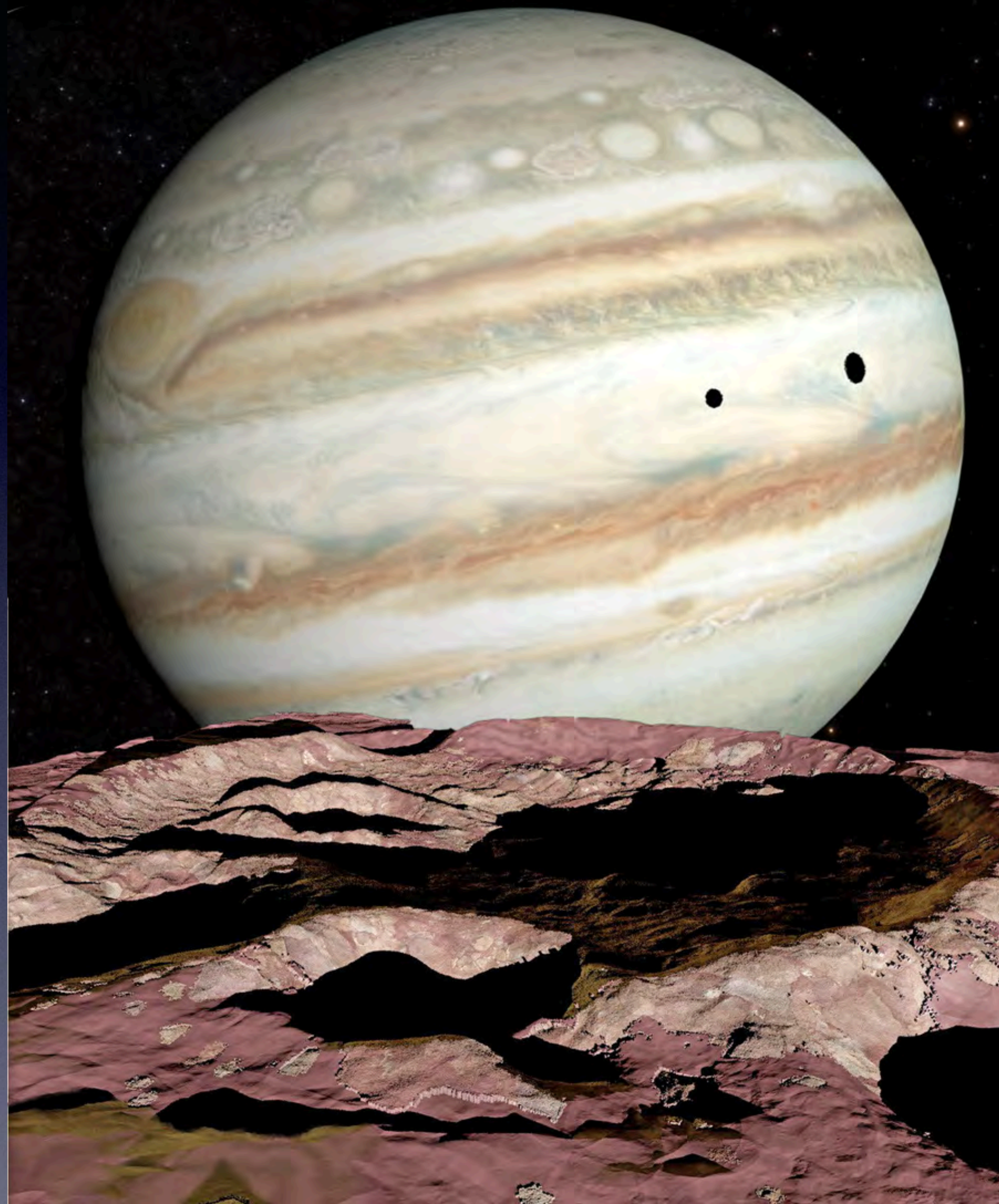
AMALTHEA
